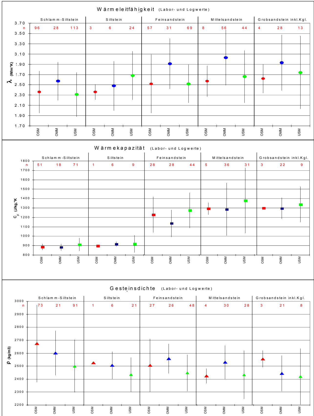
Abb. 10.9 Arithmetischer Mittelwert und Standardabweichung der Stoffwerte des Bodens im Molassebecken des Schweizerischen Mittellandes nach Leu et al. (1999). OSM: Obere Süsswassermolasse, OMM: Obere Meeressmolasse, USM: Untere Süsswassermolasse
