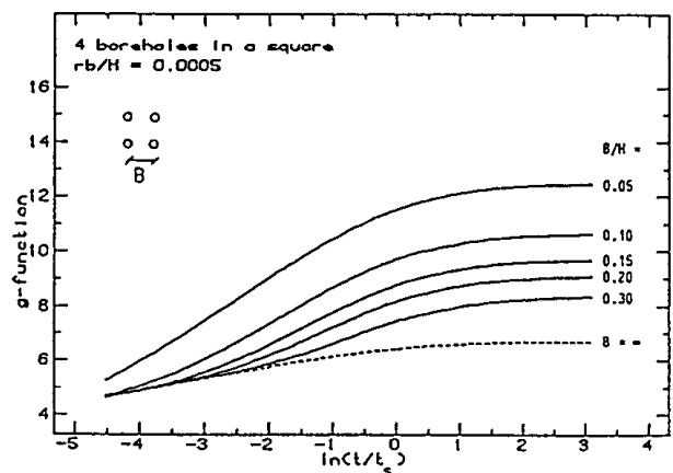
Abb. 10.10 Ausgewählte Temperatursprungantworten (g-functions) für Erdwärmesondenfelder aus Eskilson (1987)
