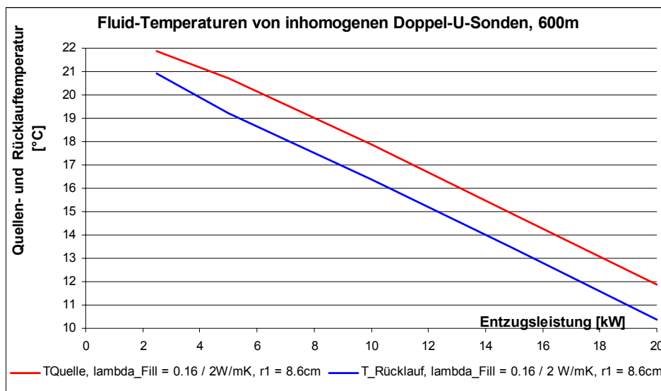
Abb. 5.16 Einfluss der Entzugsleistung auf die Fluidtemperaturen von inhomogenen Doppel-U-Sonde 50 mm mit einer Schaumzement hinterfüllung mit \lambda_{Fill} = 0.16 \text{ W/mK} in den ersten 70% der Bohrtiefe und mit einer Quarzsand hinterfüllung mit \lambda_{Fill} = 2.0 \text{ W/mK} bis auf 600m Tiefe bei 31 Tagen Dauerbetrieb (Sprungantwort). Wärmeleitfähigkeit der Erde \lambda_{Earth} = 2.6 \text{ W/mK} , Jahresdurchschnittstemperatur der Oberfläche 11°C, Temperaturgradient 3.5°C/100m, Bohrdurchmesser 17.2cm, Exzentrizität = 0.5.
