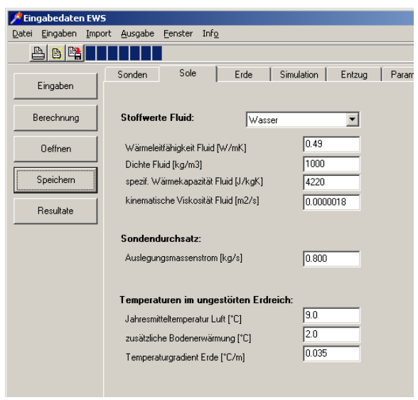
Abb. 10.6 Parameter des Sondenfluids und Temperaturen im ungestörten Erdreich
