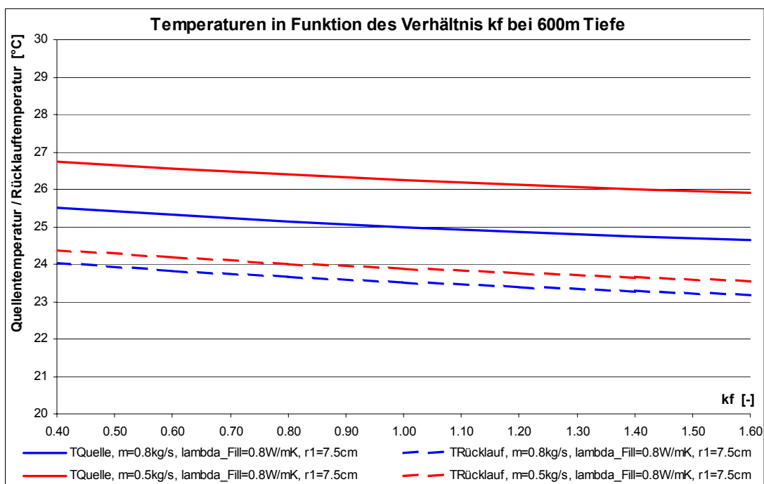
Abb. 5.23 Quellentemperaturen und Rücklaufemperaturen in Funktion des Fließgeschwindigkeitsverhältnis kf für homogene Koaxialsonden von 600m Tiefe
