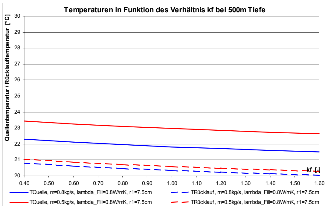
Abb. 5.22 Quellentemperaturen und Rücklaufemperaturen in Funktion des Fließgeschwindigkeitsverhältnis kf für homogene Koaxialsonden von 500m Tiefe
