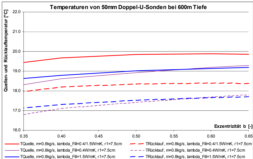
Abb. 5.13 Einfluss der Exzentrizität b auf die Quellen- und Rücklauf Temperatur der Sonde am Beispiel einer 600m tiefen Doppel-U-Sonde 50 mm mit einem Sondendurchsatz von 0.8 kg/s Wasser bei einer Entzugsleistung von 5 kW und 31 Tagen Dauerbetrieb (Sprungantwort). Wärmeleitfähigkeit der Erde \lambda_{\text{Earth}} = 2.6 \text{ W/mK} , Jahresdurchschnittstemperatur der Oberfläche 11°C, Temperaturgradient 3.5°C/100m, Bohrdurchmesser 15cm.
