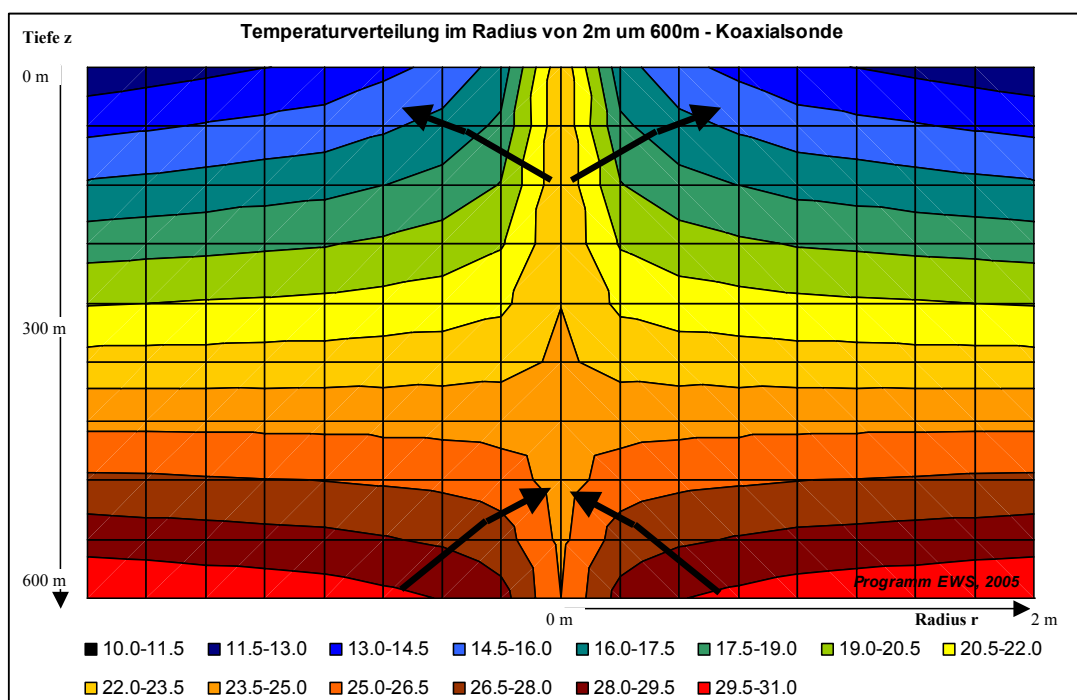
Abb. 1.1 Temperaturverteilung und Wärmefluss im Erdreich mit \lambda_{Erde} = 2.6 \text{ W/mK} um eine 600m tiefe Koaxialsonde mit Sondendurchsatz = 0.8 kg/s, Wärmeentzug 5kW nach 31 Tagen Dauerentzug. Oberflächentemperatur T_{mo} = 11^\circ\text{C} mit einem Temperaturgradienten \Delta T_{Grad} = 0.035 \text{ K/m} . Die Berechnung wurde durchgeführt mit dem Programm EWS.
