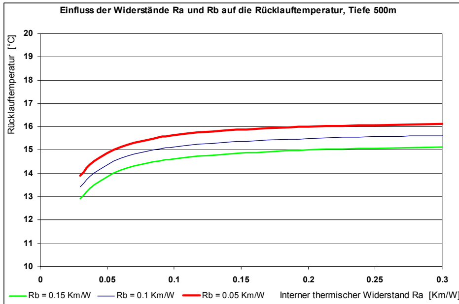
Abb. 5.3 Einfluss von Ra und Rb auf die Rücklauftemperatur der Sonde am Beispiel einer 500m tiefen Doppel-U-Sonde 50 mm mit einem Sondendurchsatz von 0.8 kg/s Wasser bei einer Entzugsleistung von 5 kW und 31 Tagen Dauerbetrieb (Sprungantwort). Wärmeleitfähigkeit der Erde \lambda_{Earth} = 2.6 \text{ W/mK} , Jahresdurchschnittstemperatur der Oberfläche 11°C, Temperaturgradient 3.5°C/100m, Bohrdurchmesser 15cm.
