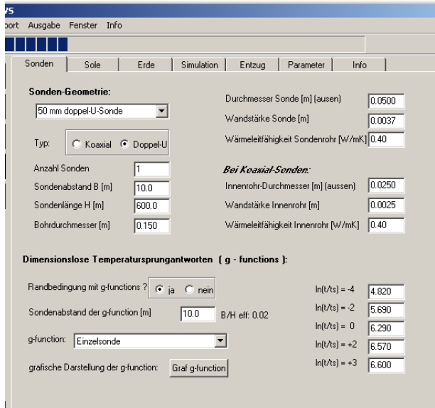
Abb. 10.5 Geometrische Sondenparameter und verwendete g-function
