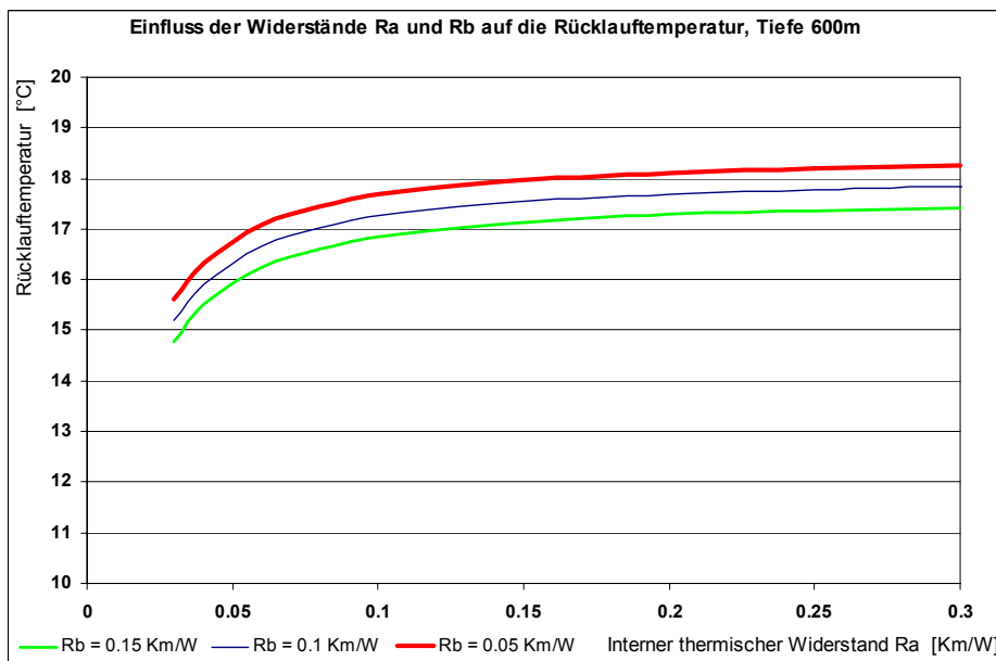
Abb. 5.4 Einfluss von Ra und Rb auf die Quelltemperatur der Sonde am Beispiel einer 600m tiefen Doppel-U-Sonde 50 mm mit einem Sondendurchsatz von 0.8 kg/s Wasser bei einer Entzugsleistung von 5 kW und 31 Tagen Dauerbetrieb (Sprungantwort). Wärmeleitfähigkeit der Erde \lambda_{Earth} = 2.6 \text{ W/mK} , Jahresdurchschnittstemperatur der Oberfläche 11°C, Temperaturgradient 3.5°C/100m, Bohrdurchmesser 15cm.
