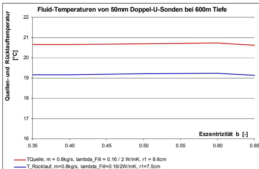
Abb. 5.14 Quellen- und Rücklauf Temperatur des Sondenfluids einer 600m tiefen Doppel-U-Sonde 50 mm mit einer Schaumzementhinterfüllung mit \lambda_{Fill} = 0.16 W/mK in den ersten 420m und mit einer Quarzsandhinterfüllung mit \lambda_{Fill} = 2.0 W/mK bis auf 600m Tiefe. Sondendurchsatz 0.8 kg/s, Entzugsleistung 5 kW und 31 Tagen Dauerbetrieb (Sprungantwort). Wärmeleitfähigkeit der Erde \lambda_{Earth} = 2.6 W/mK, Jahresdurchschnittstemperatur der Oberfläche 11°C, Temperaturgradient 3.5°C/100m, Bohrdurchmesser 17.2cm.
