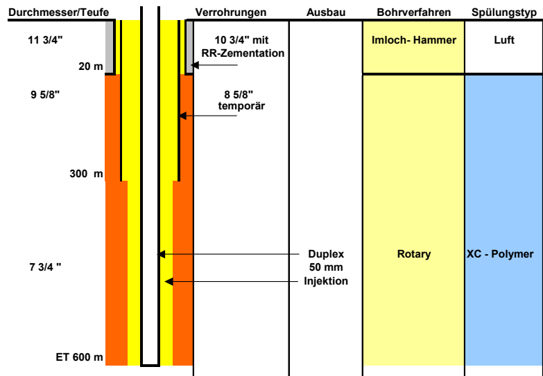
Abb. 6.4 Vorschlag Hr. Berli (Foralith AG) für Bohr- und Verrohrungsschema für eine 600m tiefe, 50mm Doppel-U-Sonde bei unbekanntem Bohrverhältnissen.
