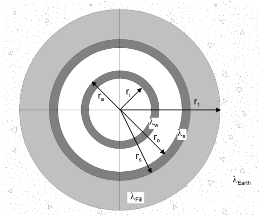
Abb. 3.9 Bezeichnungen an der Koaxialsonde
