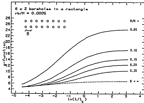
Abb. 10.10 Ausgewählte Temperatursprungantworten (g-functions) für Erdwärmesondenfelder aus Eskilson (1987)
