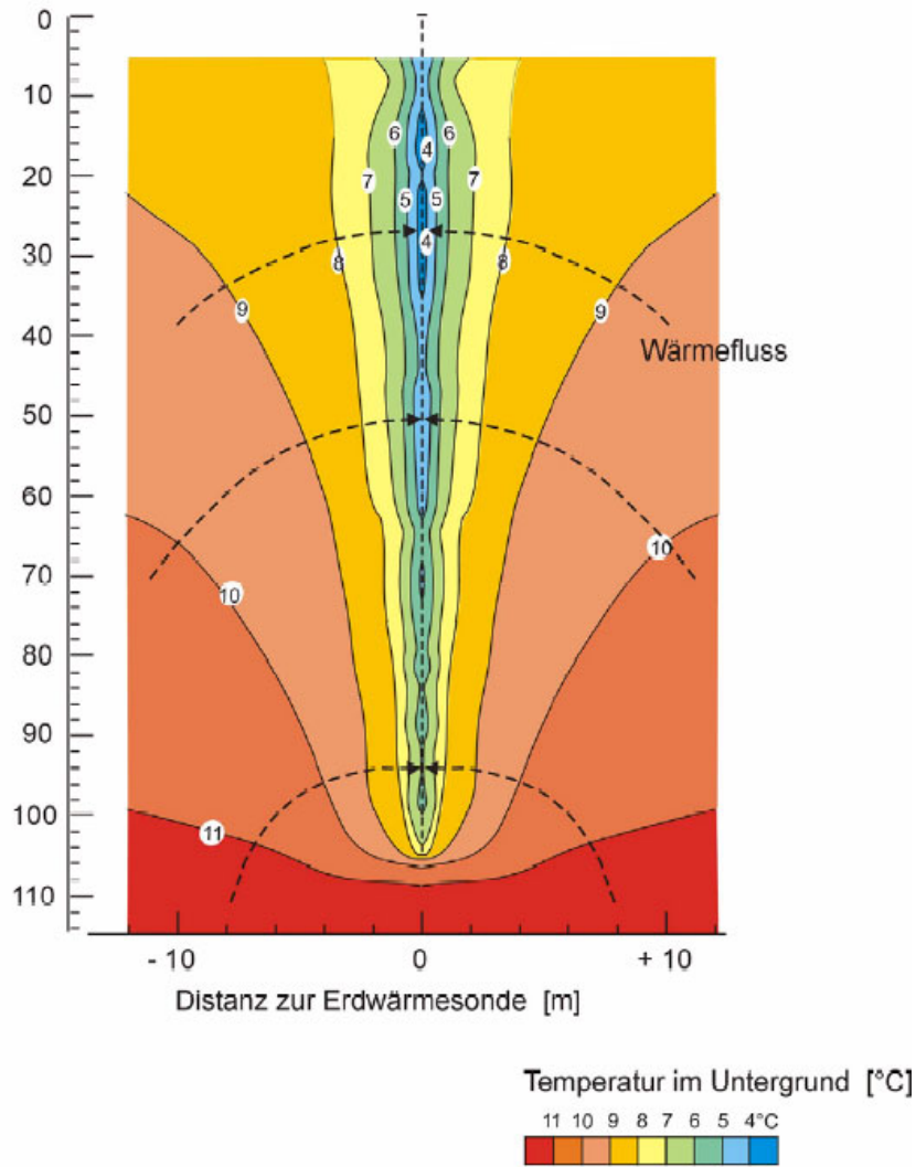
Abb. 2.3 Wärmeflusslinien beim Wärmeentzug, Anlage Elgg am kältesten Wintertag, berechnet mit dem Programm Cosond [Eugster, 1998]. Zu beachten ist die unterschiedliche Skala in x- und z-Richtung.
