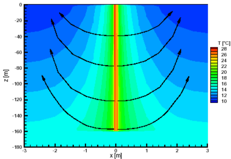
Abb. 2.4 Wärmeflusslinien bei einer 160m tiefen Erdwärmesonde bei einem Response-Test mit Wärmeeintrag, berechnet mit dem Programm Fracture [Signorelli, 2004].
