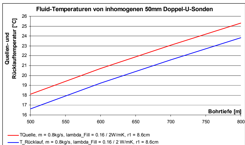
Abb. 5.15 Fluidtemperaturen von inhomogenen Doppel-U-Sonde 50 mm mit einer Schaumzementhinterfüllung mit \lambda_{Fill} = 0.16 W/mK in den ersten 70% der Bohrtiefe und mit einer Quarzsandhinterfüllung mit \lambda_{Fill} = 2.0 W/mK bis auf 600m Tiefe. Sondendurchsatz 0.8 kg/s, Entzugsleistung 5 kW und 31 Tagen Dauerbetrieb (Sprungantwort). Wärmeleitfähigkeit der Erde \lambda_{Earth} = 2.6 W/mK, Jahresdurchschnittstemperatur der Oberfläche 11°C, Temperaturgradient 3.5°C/100m, Bohrdurchmesser 17.2cm.
