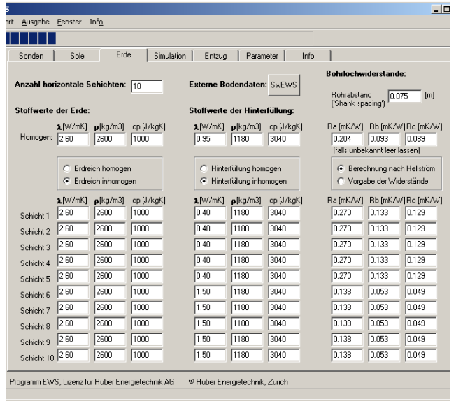
Abb. 10.7 Stoffwerte des Bodens, der Hinterfüllung und Bohrlochwiderstände
